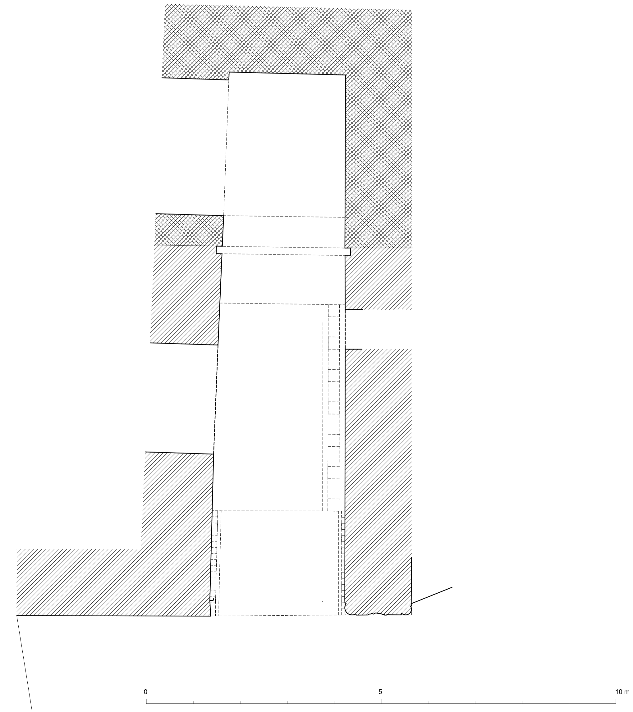
TARIFA. PUERTA DE LA ALMEDINA ANTONIO ALMAGRO / arq. Junio 2022
