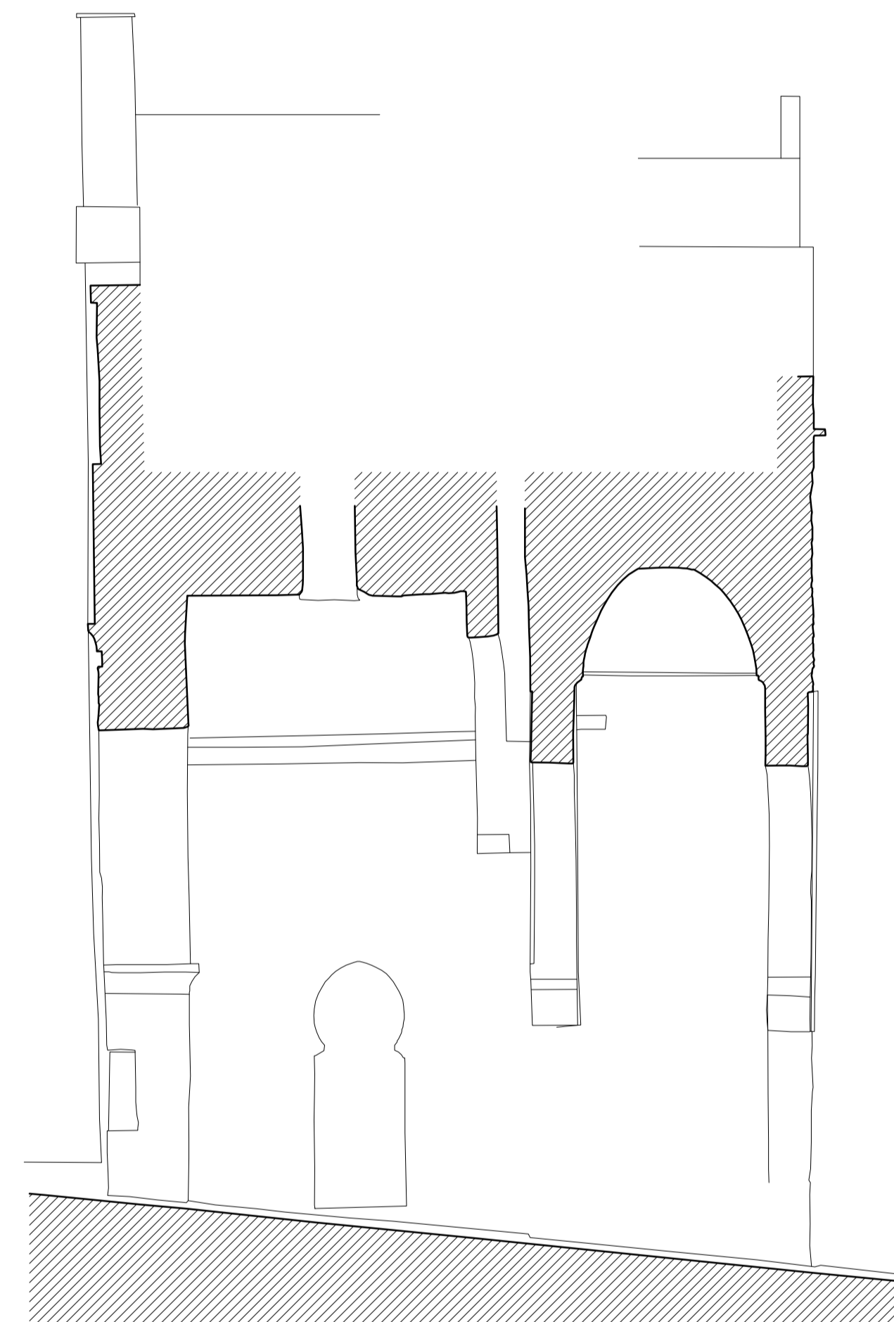
0 5 10 m RECINTO AMURALLADO DE TARIFA ( Cádiz ) . PUERTA DE JEREZ A. ALMAGRO / arq. RABASF JUNIO 2022
