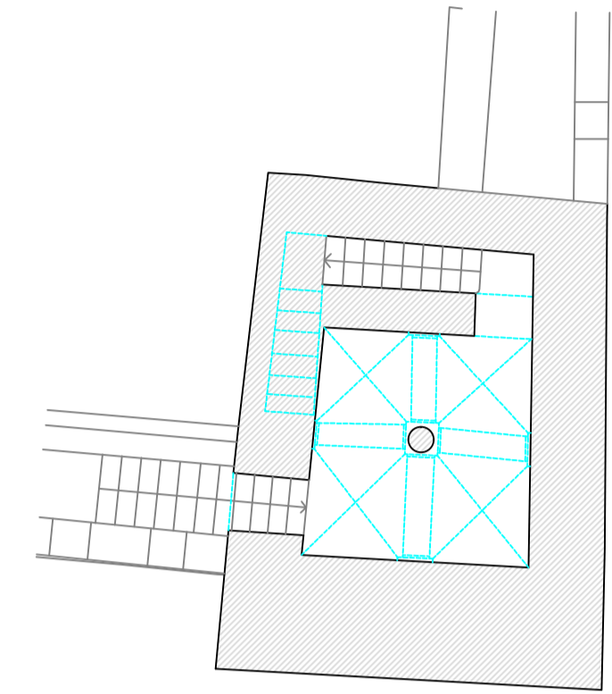
PLANTA DE LA CAMARA
