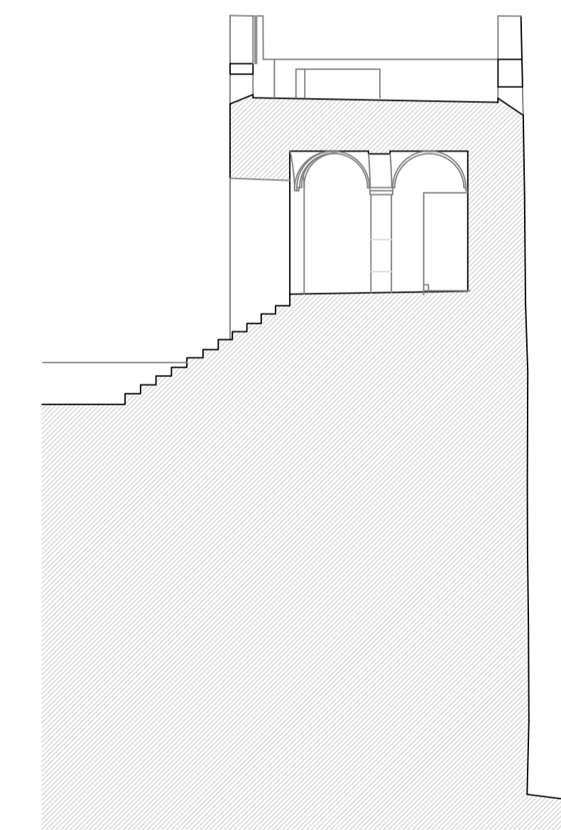
SECCION
