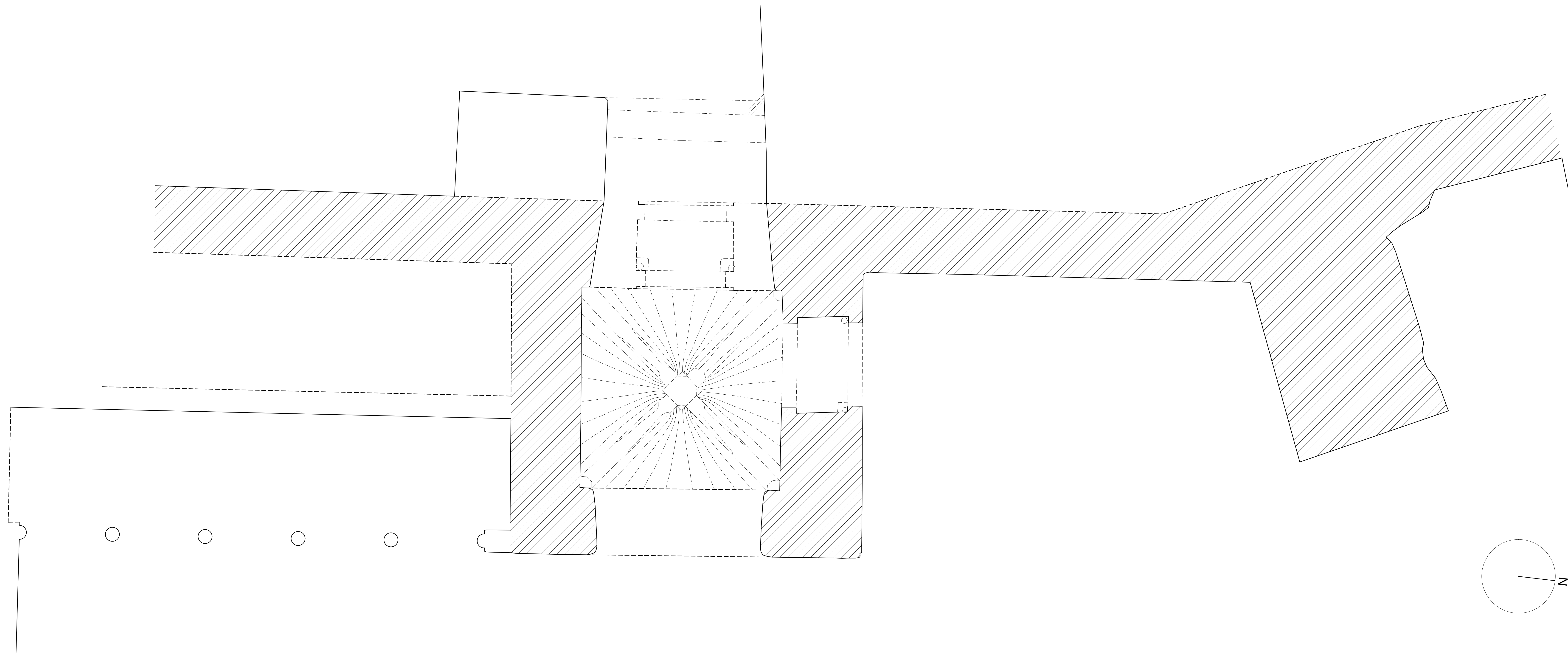
PLANTA
