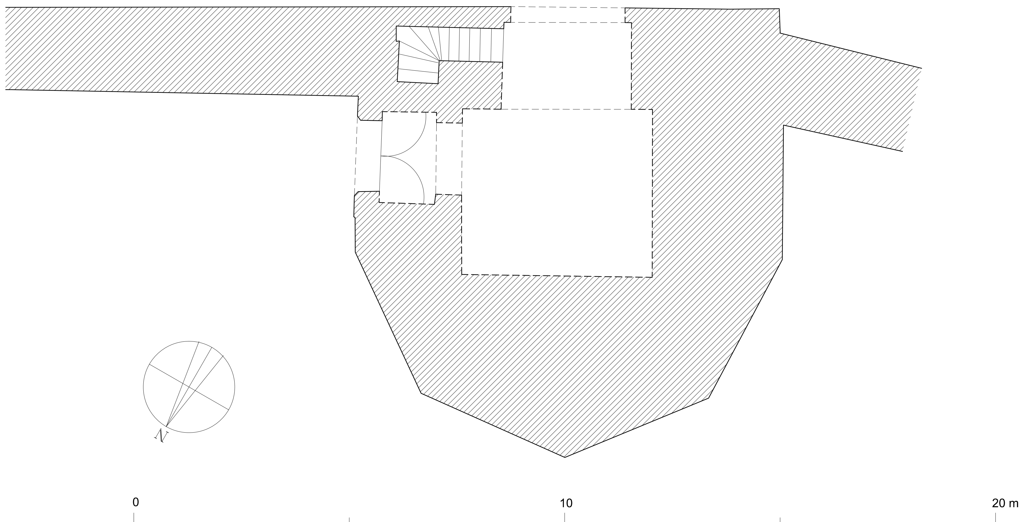
RECINTO AMURALLADO DE PALMA DEL RÍO (CÓRDOBA) . PUERTA NORTE HIPÓTESIS A. ALMAGRO y J. RABASF OCTUBRE 2022
