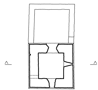
Intradós Norte
