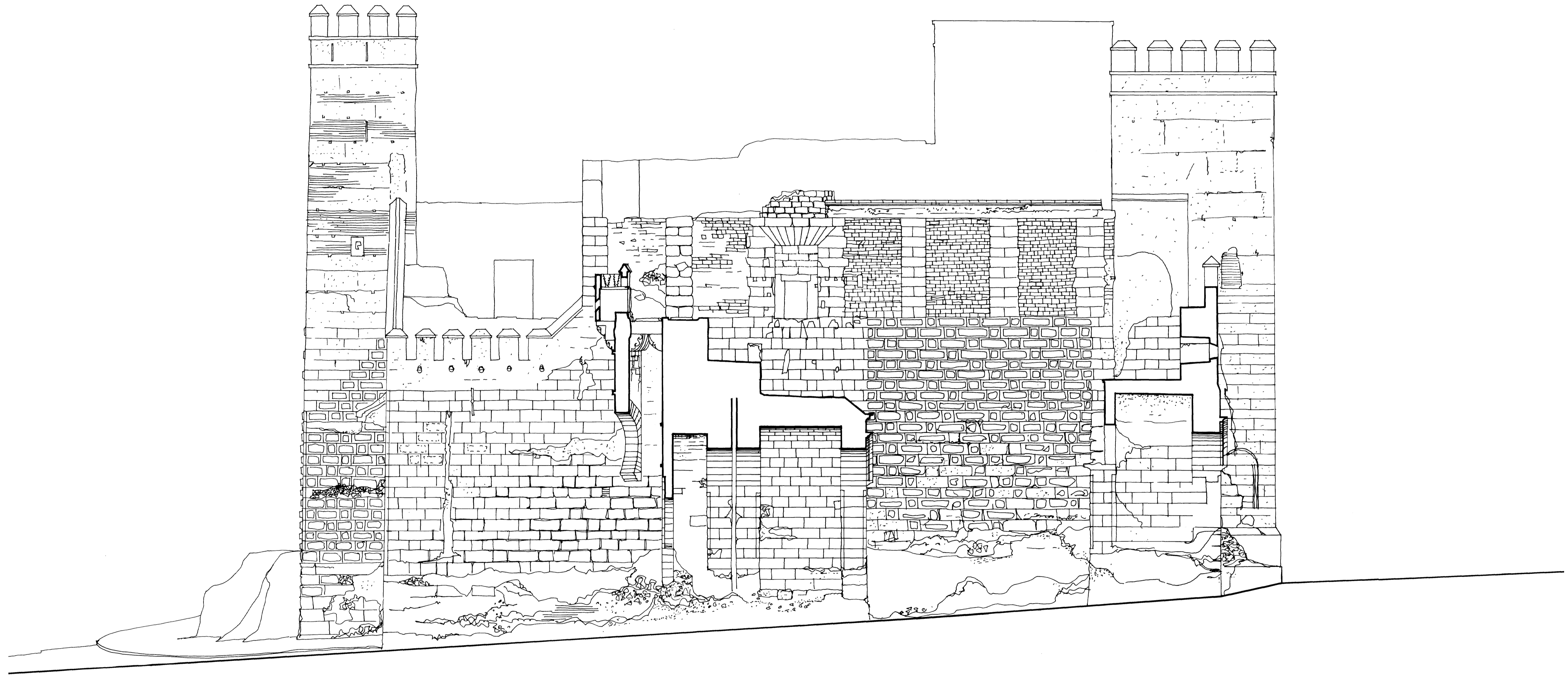
ALZADO SUR Y ECCIÓN POR PUERTA
