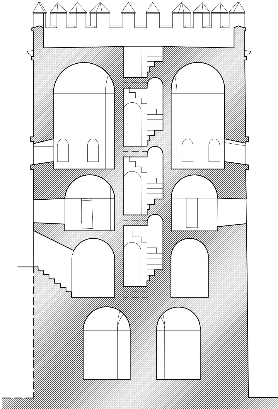
SECCION HIPOTESIS TORRE ALMOHADE
