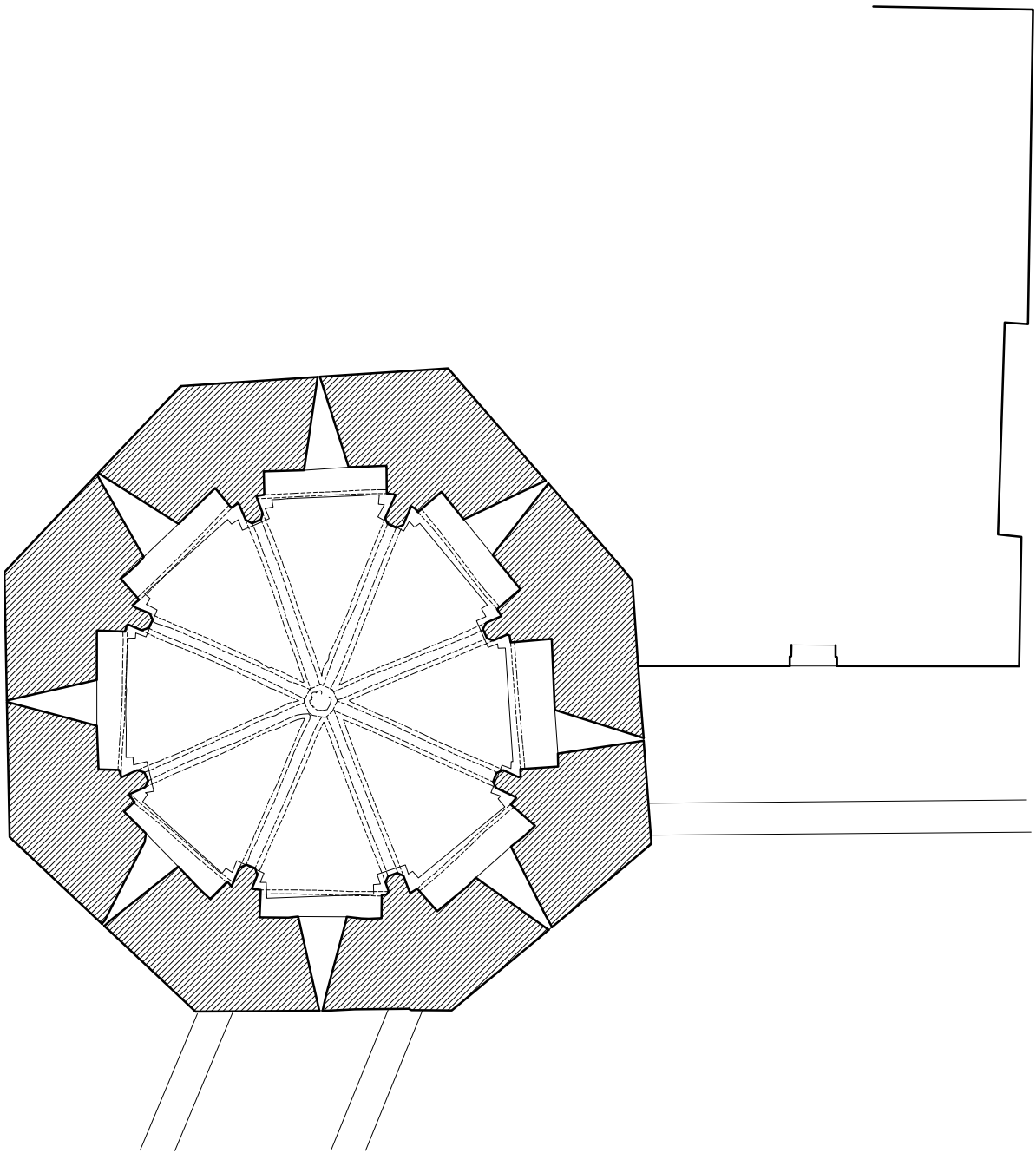
PLANTA NIVEL 3
