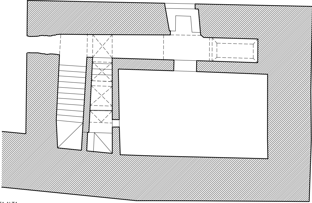
PLANTA ALTA
