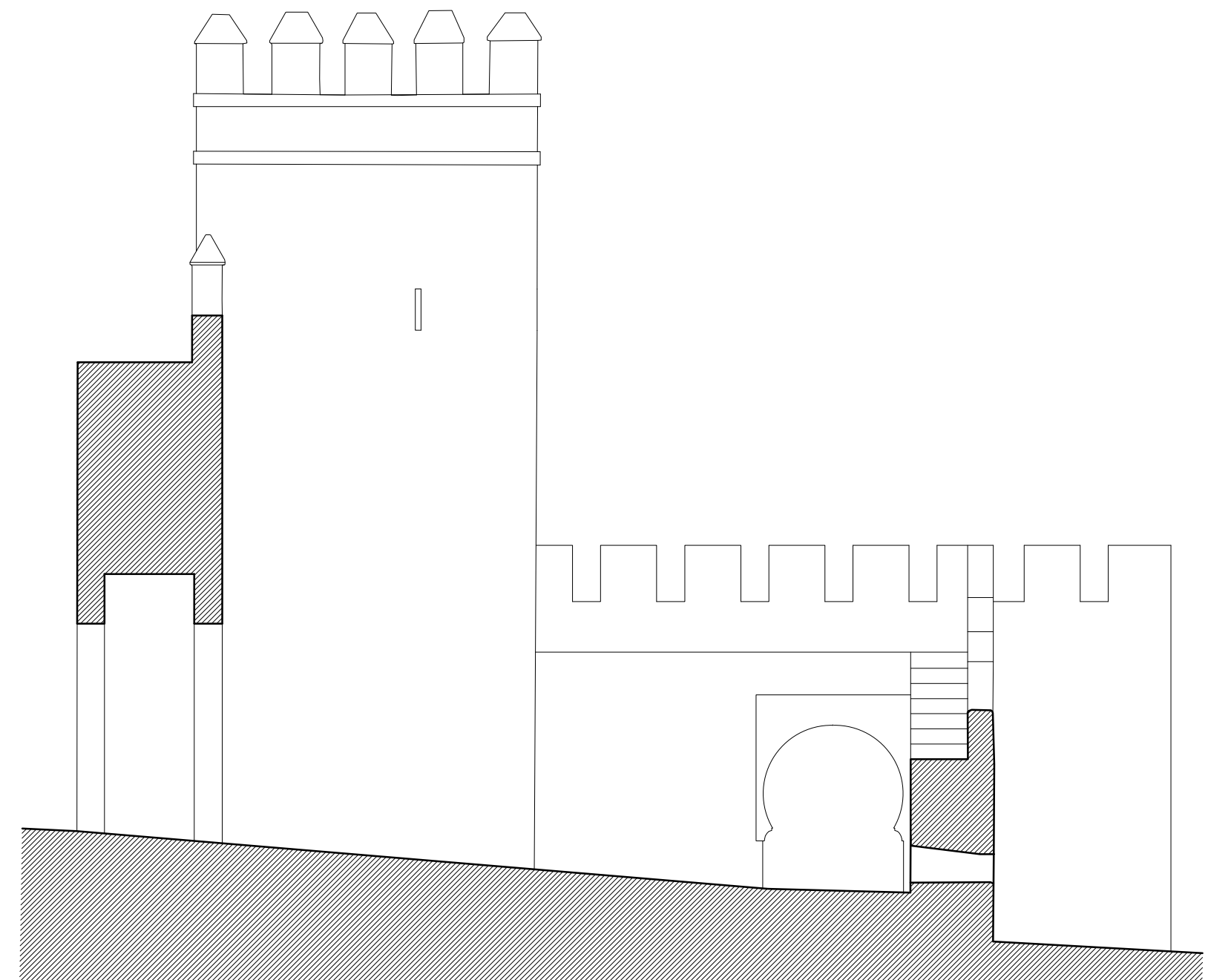
SECCION POR LA PUERTA
