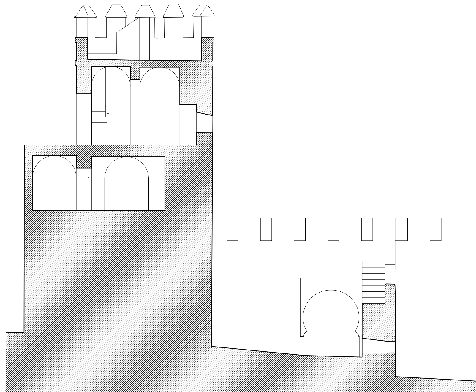
SECCION POR LA TORRE
