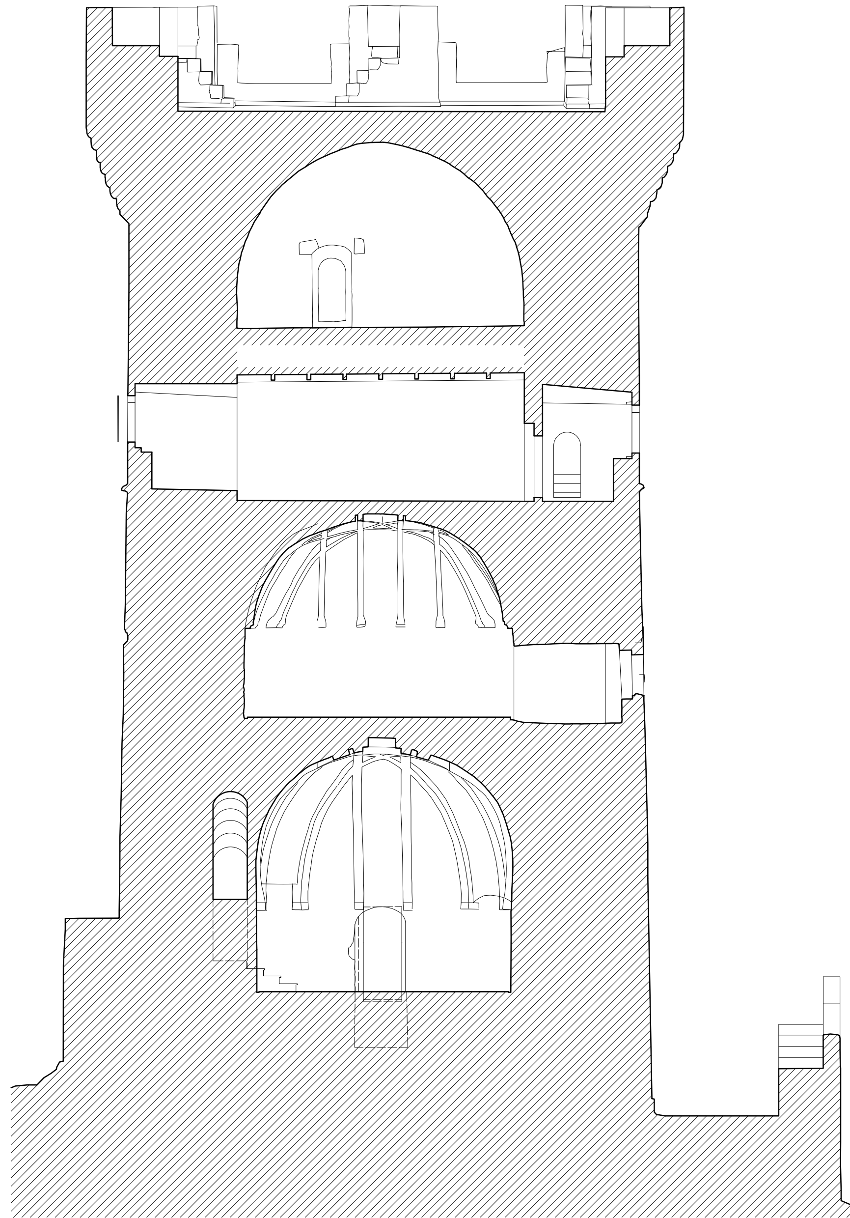
SECCION N-S
