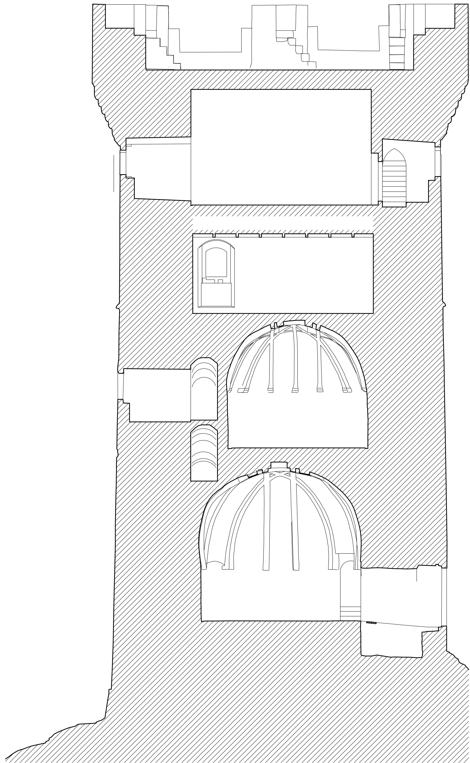
SECCION O-E
