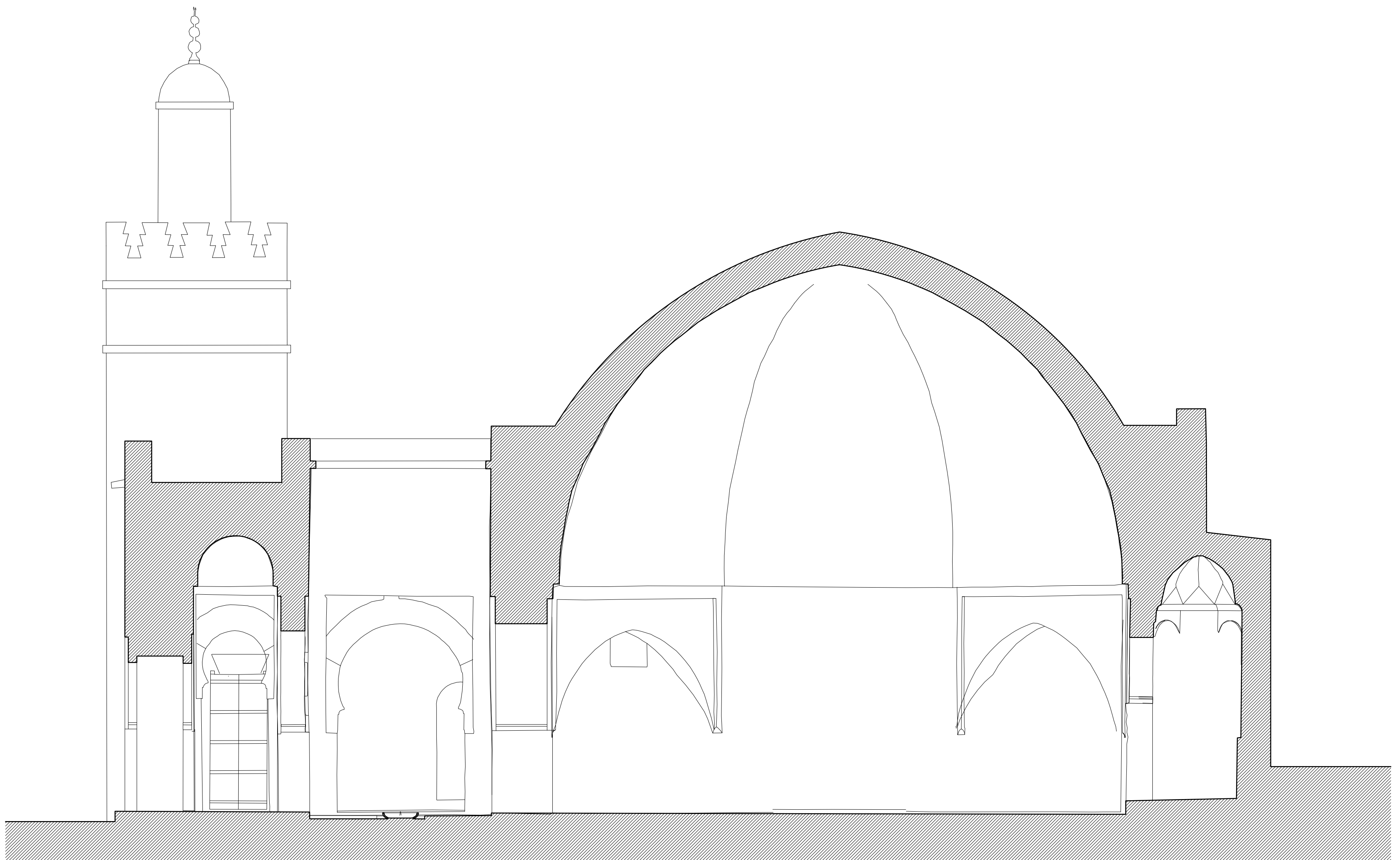
MEZQUITA DEL ALCAZAR DE JEREZ DE LA FRONTERA (CÁDIZ) A. ALMAGRO / arq. RABASF
