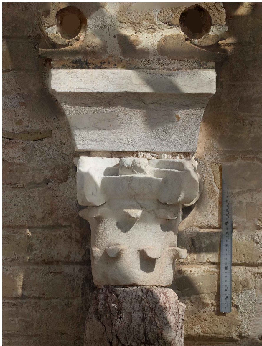
TORRE DE LA GIRALDA. SEVILLA. FACHADA OESTE. CAPITEL O302
