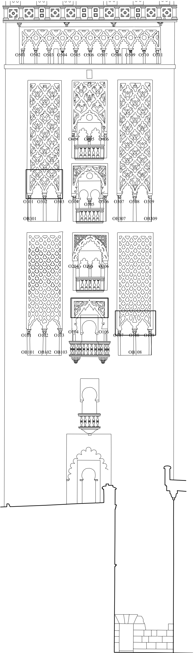
PLANO INDICE DE LOS CAPITELAS DEL ALZADO OESTE DE LA GIRALDA
