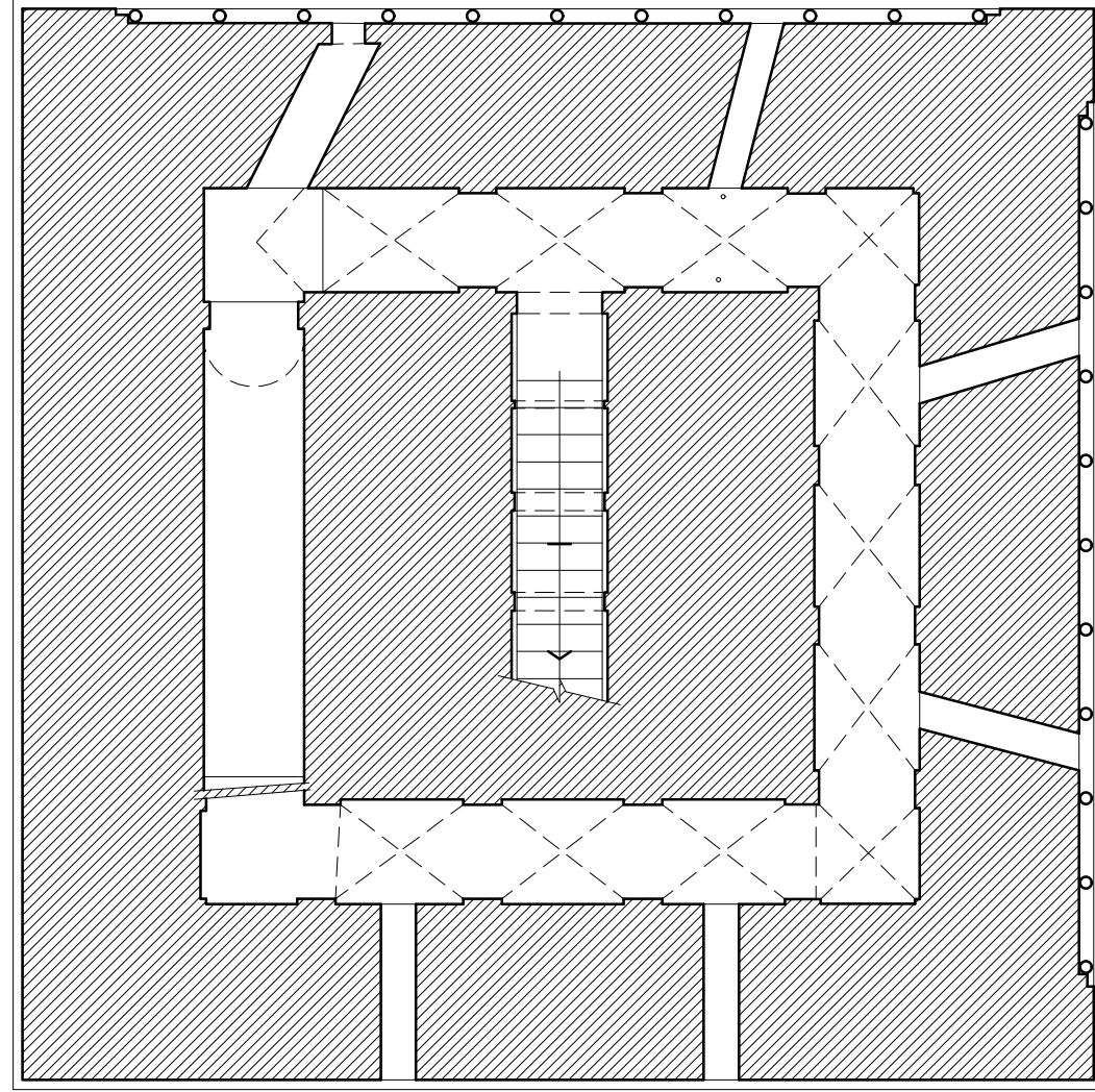
SECCIÓN ALMINAR NIVEL 8
