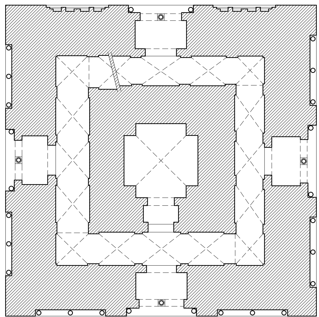
SECCIÓN ALMINAR NIVEL 6
