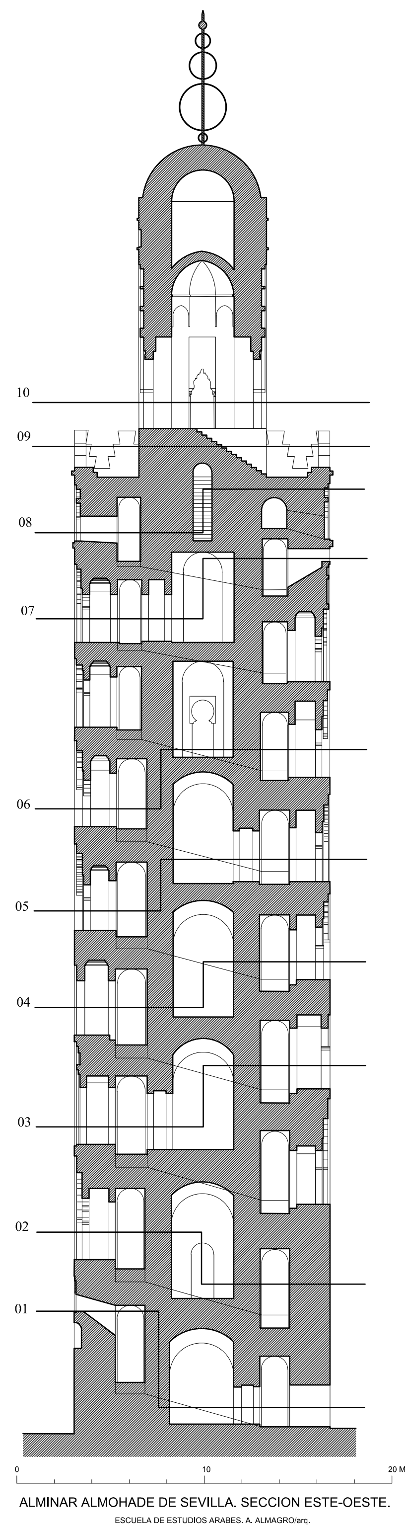
ALMINAR ALMOHADE DE SEVILLA. SECCION ESTE-OESTE. ESQUEMA DE ESTUdios ARABES. AL ALMAGRO/arg.
