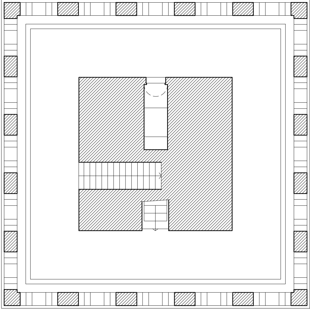
SECCIÓN ALMINAR NIVEL 9
