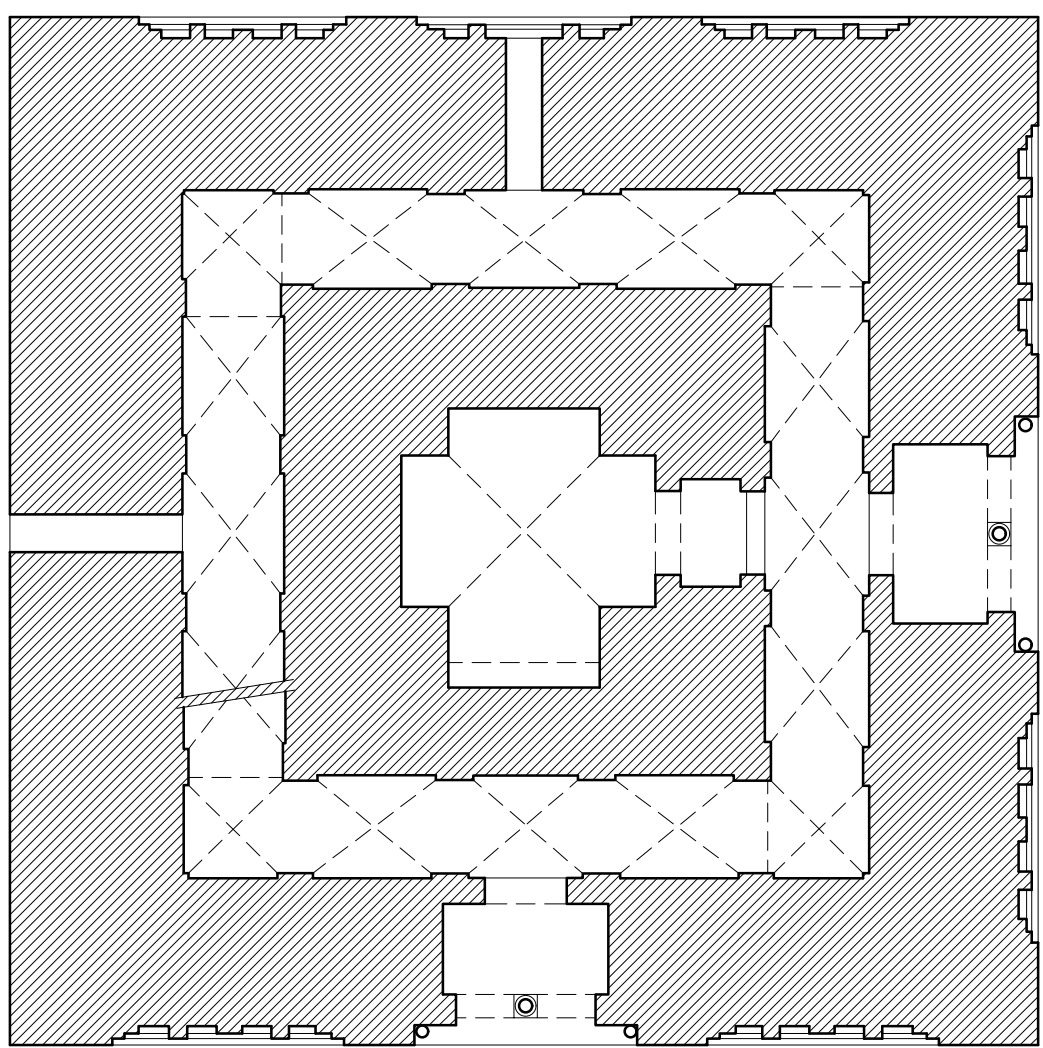
SECCIÓN ALMINAR NIVEL 7
