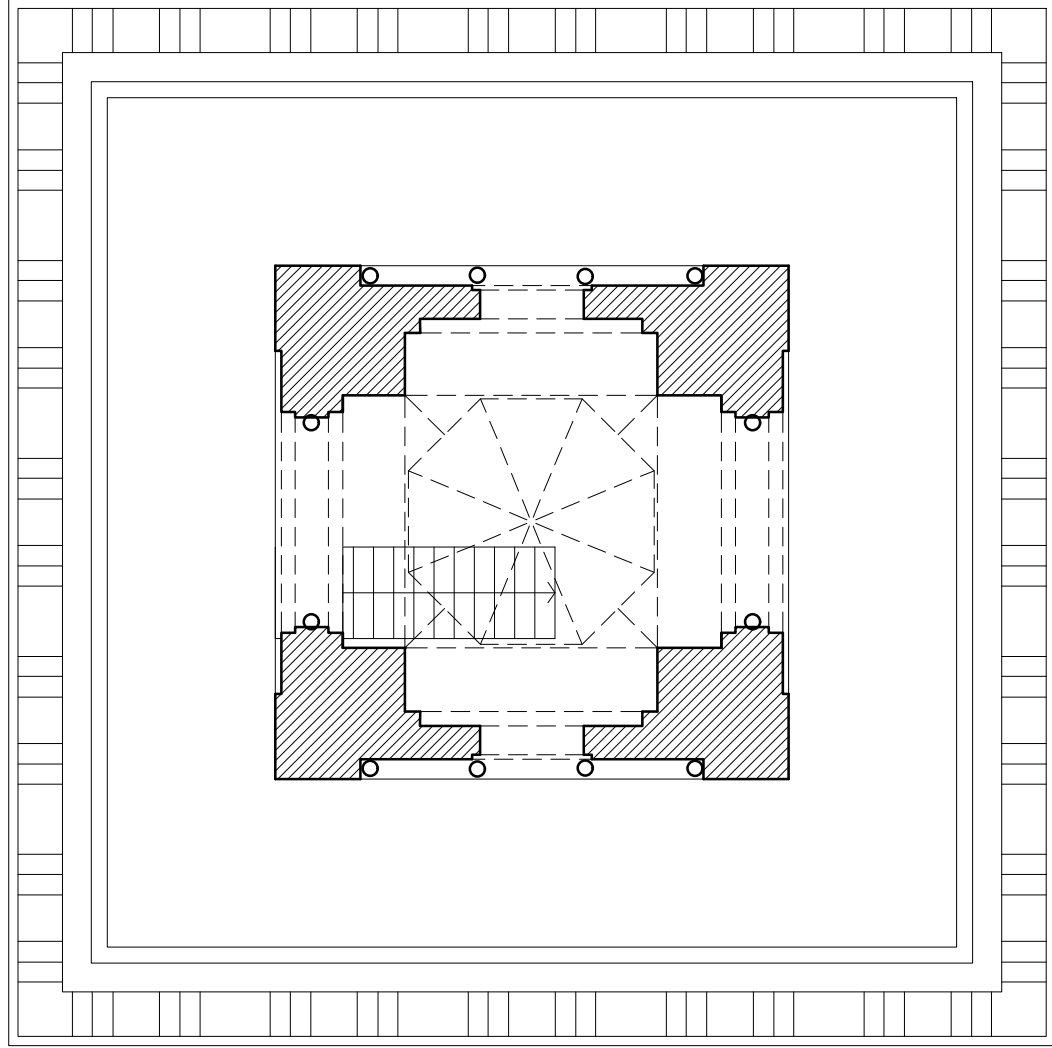
SECCIÓN ALMINAR NIVEL 10
