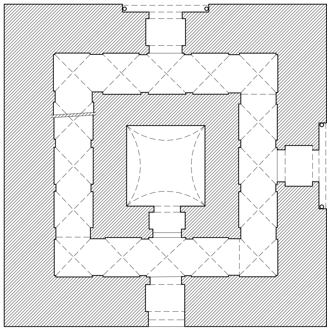
SECCIÓN ALMINAR NIVEL 2
