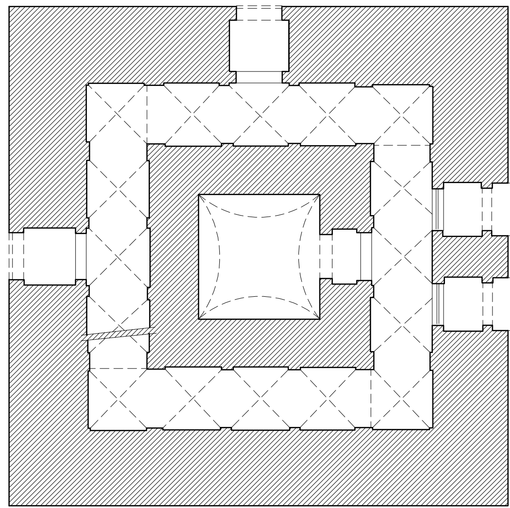
SECCIÓN ALMINAR NIVEL 3
