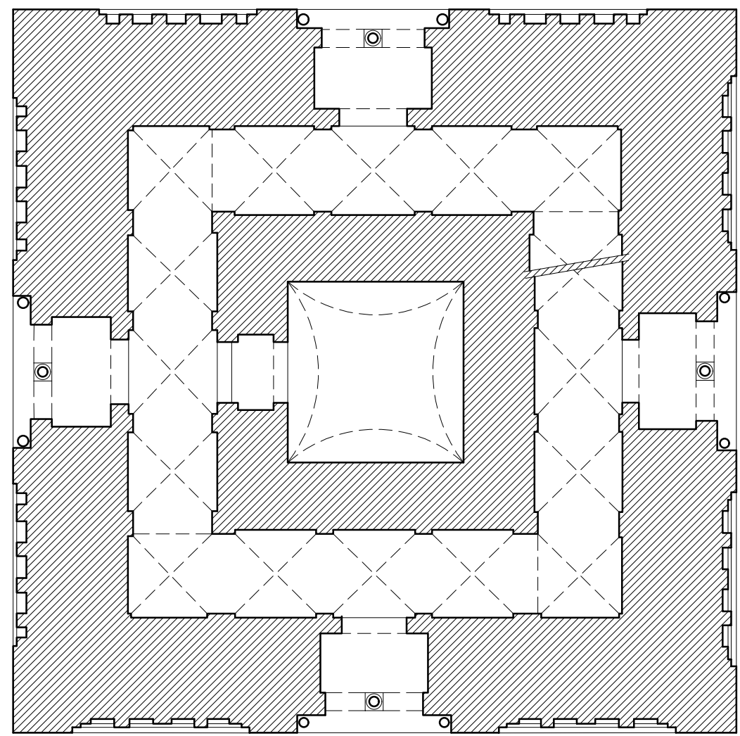
SECCIÓN ALMINAR NIVEL 5
