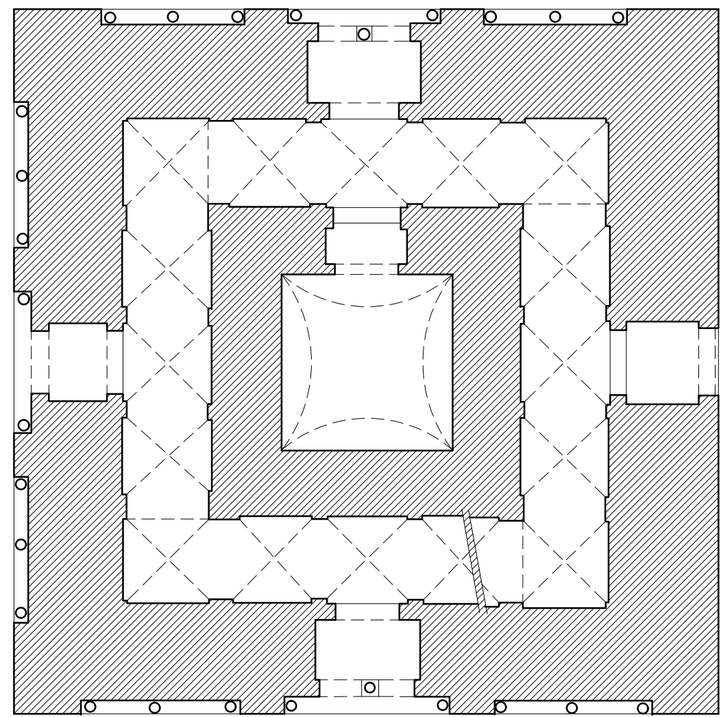
SECCIÓN ALMINAR NIVEL 4
