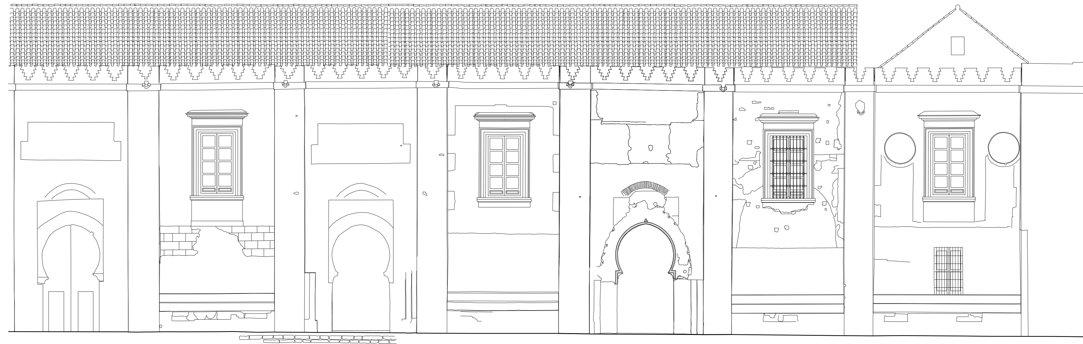
ALZADO EXTERIOR ESTE
