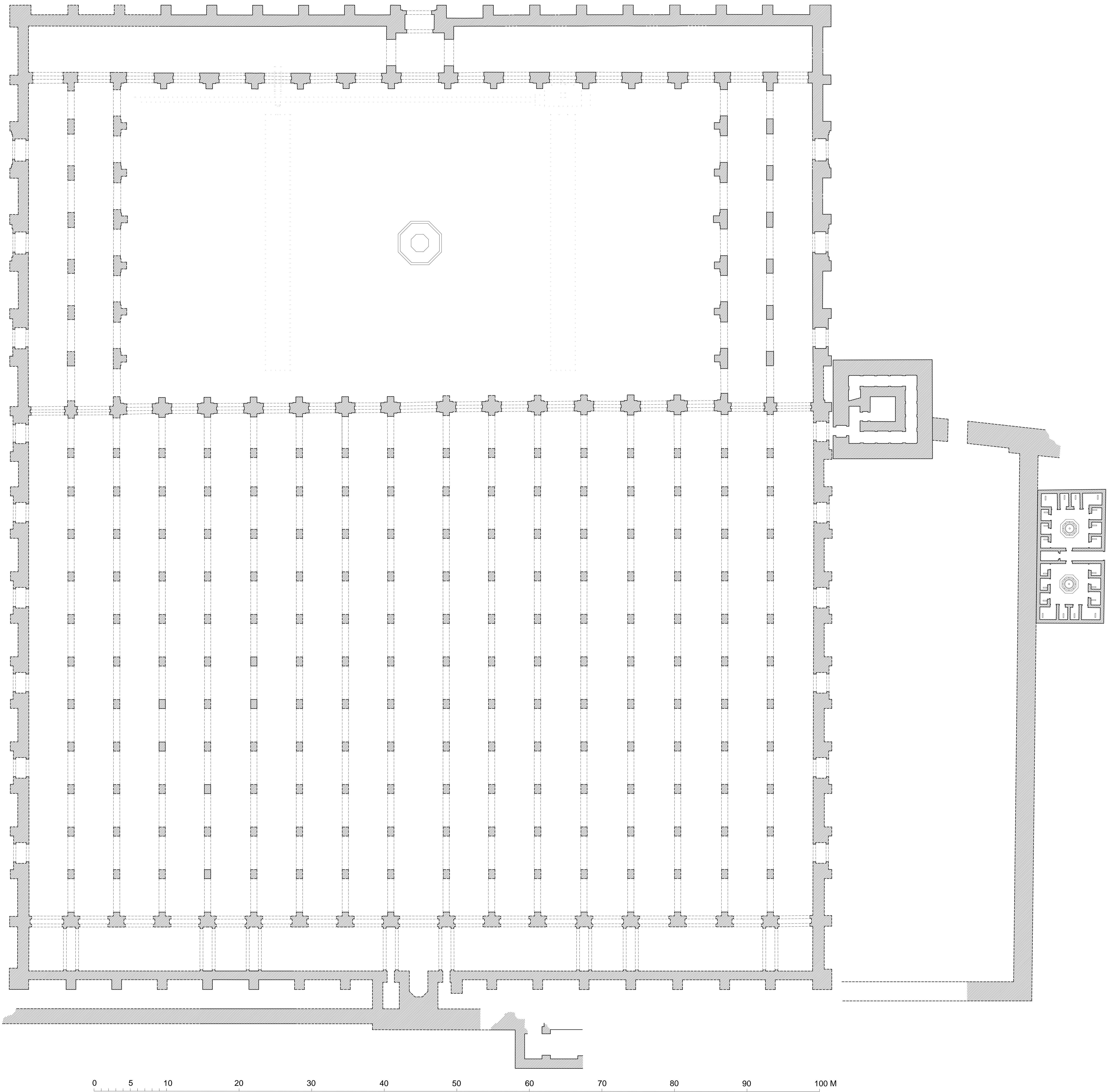
MEZQUITA ALMOHADE DE SEVILLA. PLANTA.
