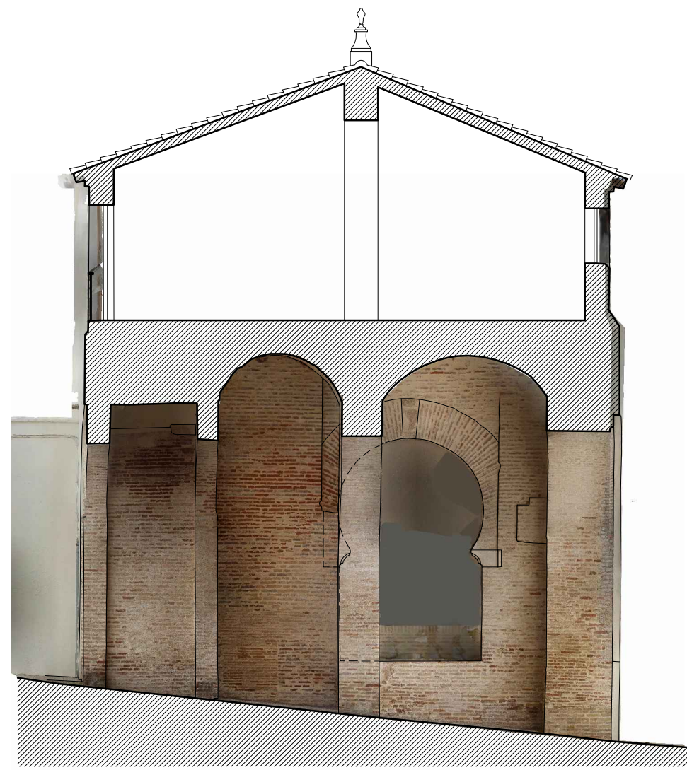
SECCION N-S
