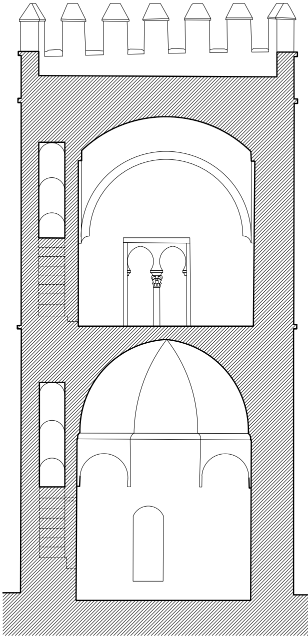
SECCION N-S
