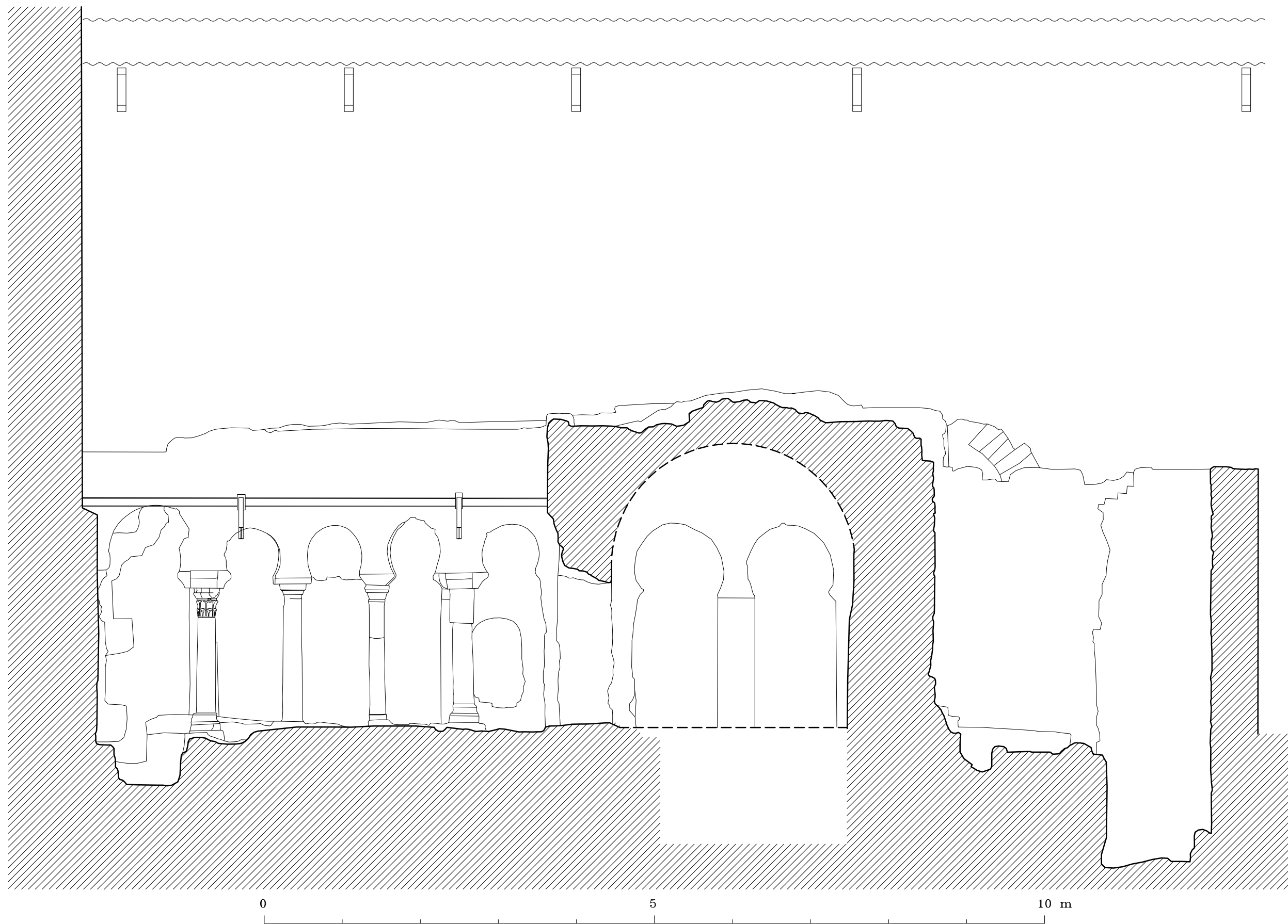
HAMMAM DEL BARRIO DE SAN PEDRO. CORDOBA. SECCION S-N HACIA OESTE
