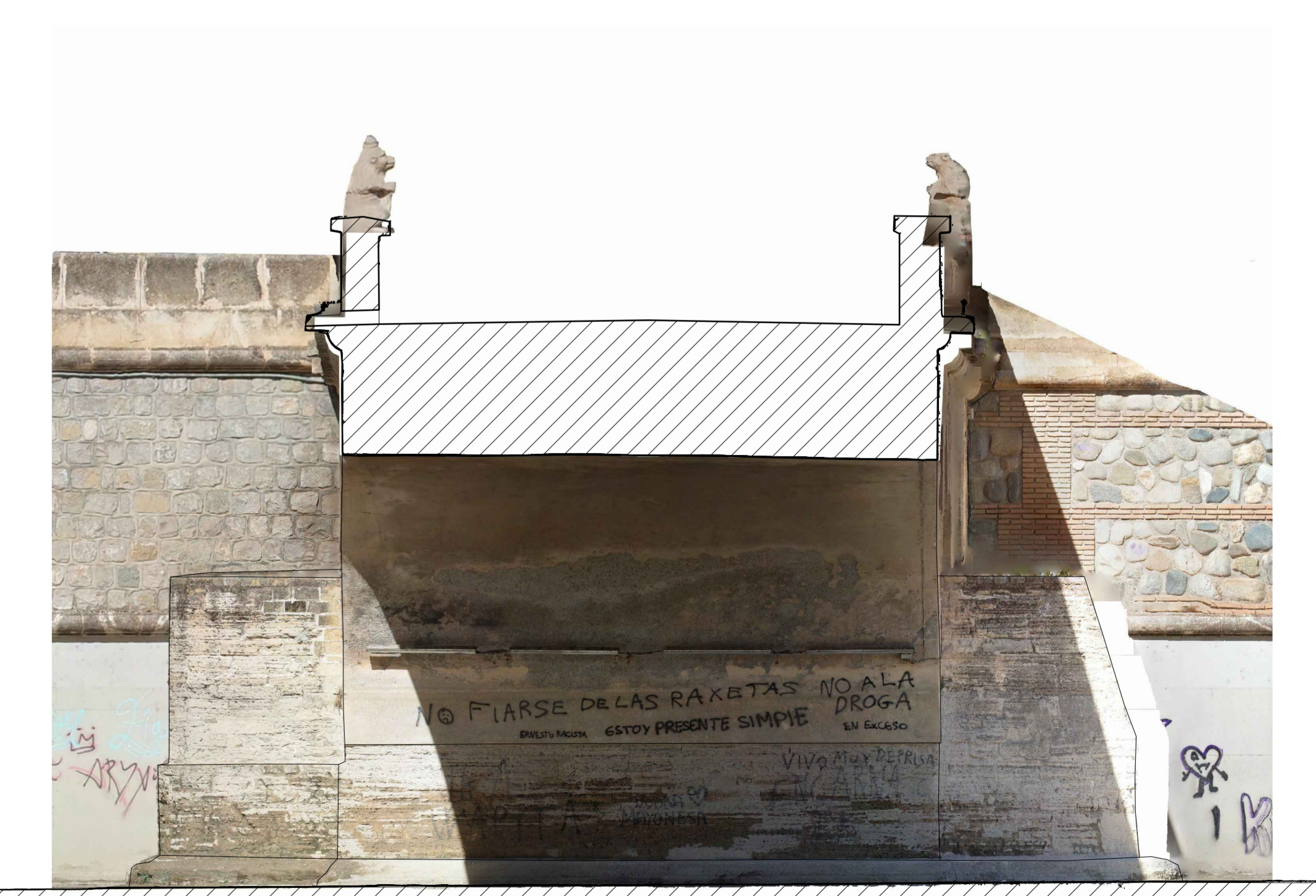
SECCION POR VANO CENTRAL
