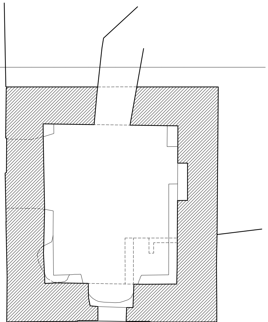
Planta nivel 1
